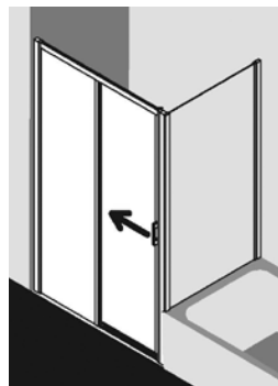
B Wanneneinbaumaß (WE) mit FORMAT Pro 2.0 Seitenwand verkürzt auf Badewanne
