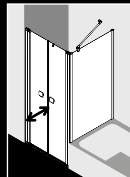
C Wanneneinbaumaß (WE) Seitenwand verkürzt auf Badewanne
