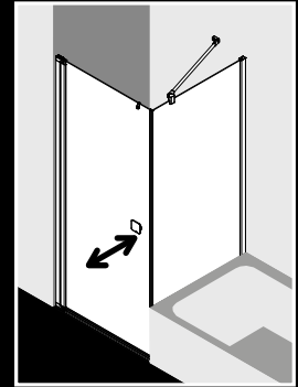
C Wanneneinbaumaß (WE) Seitenwand verkürzt auf Badewanne
